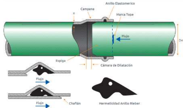
Tubería PVC Alcantarillado Sanitario Serie Inglesa
